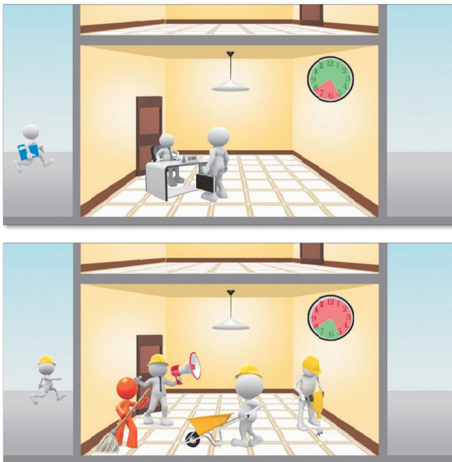
Caso b): interferenza spaziale (ma non temporale)
